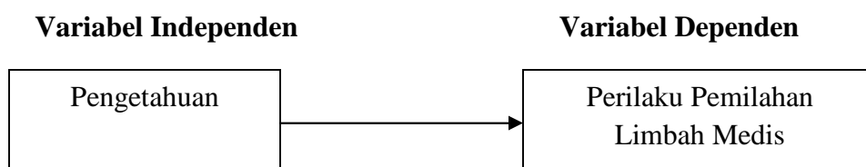
Gambar 2.1 Kerangka Berpikir
